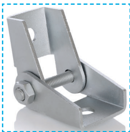
پایه پروفیل مفصلی سبک HBAS
