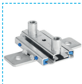
پایه اسلایدر دابل SLDO
